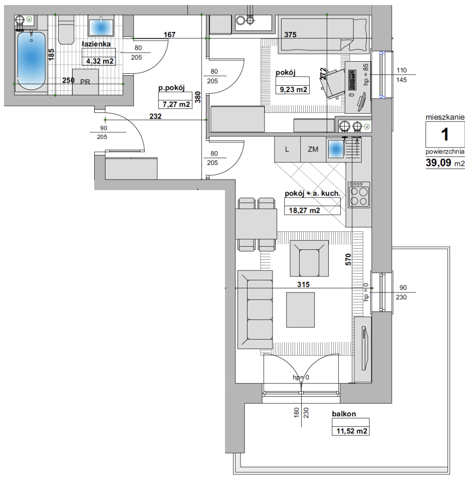
Rzut parteru
