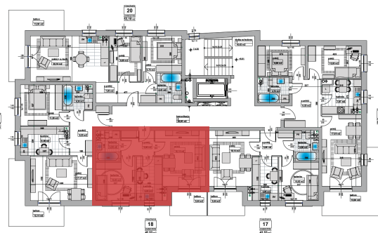
Rzut piętra
