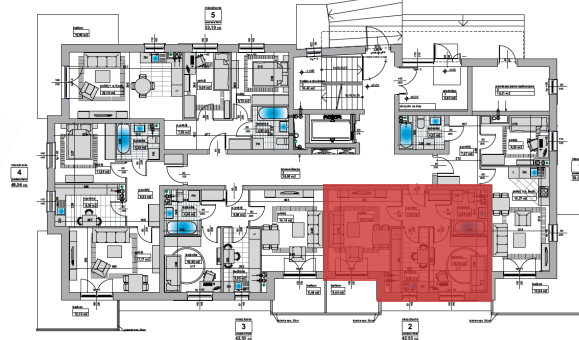
Rzut parteru
